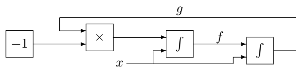
FIGURE 1 – Un GPAC engendrant les fonctions f(x) = \cos(x) et g(x) = \sin(x)
