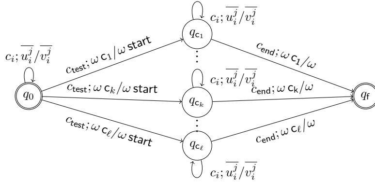
Fig. 4. Automaton \mathcal{A}_{\text{CONST}}^P
